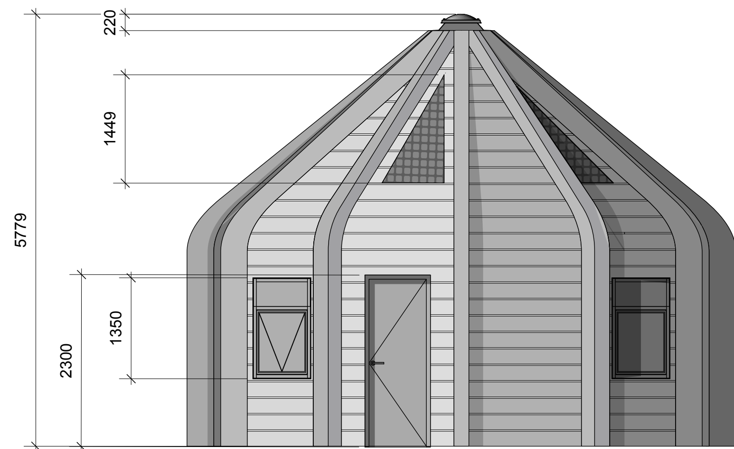
GEVEL VOOR
