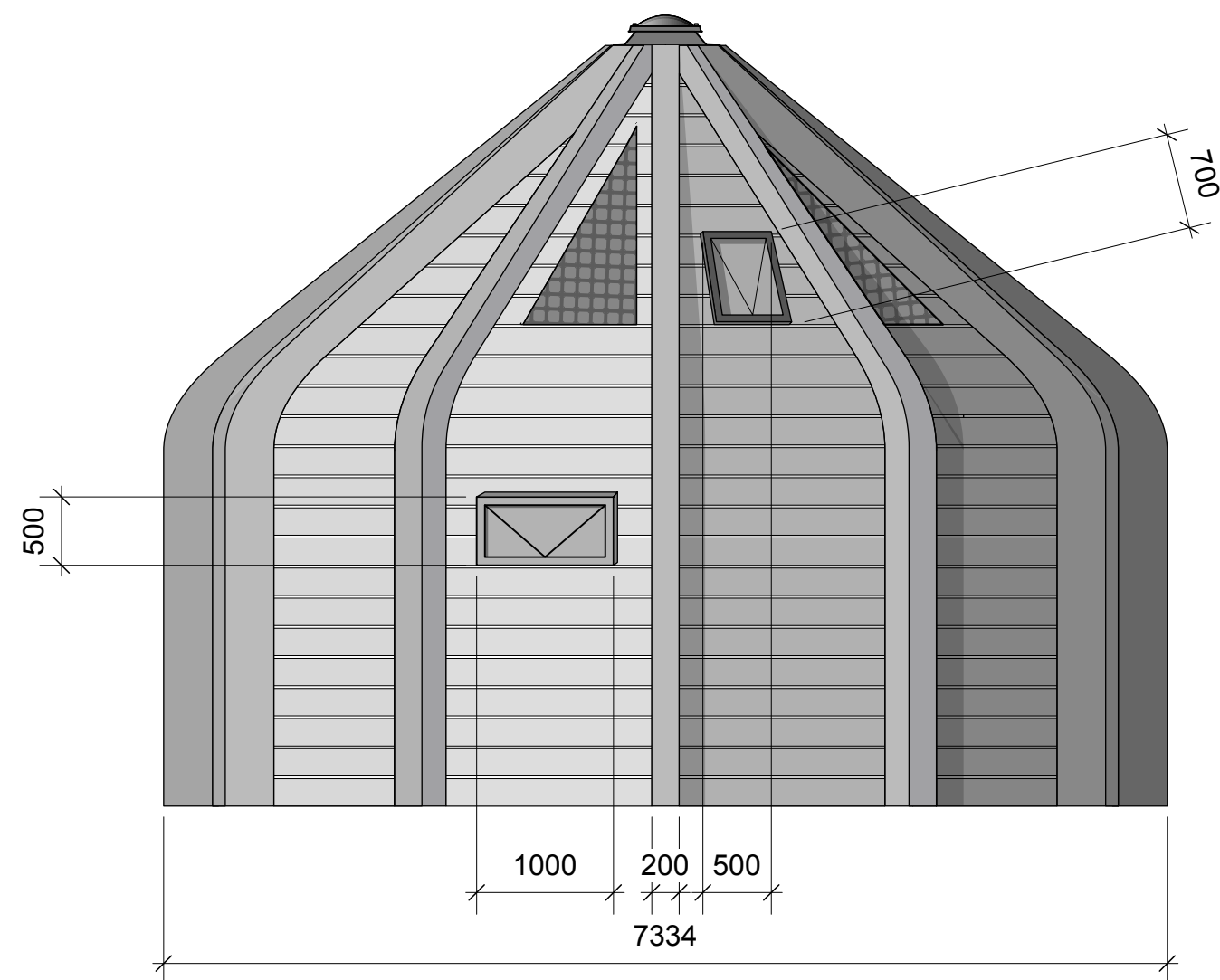
GEVEL ACHTER
